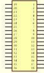
CON AT36-62
