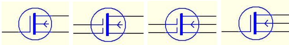
MOSFET-N1—MOSFET-N4
