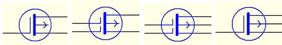
MOSFET-P1—MOSFET-P4
